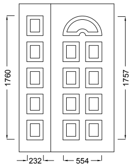
Καίτη/Transom
